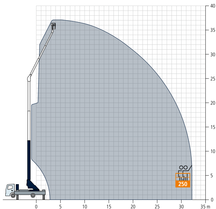
Bügelkorb PK 250-1
