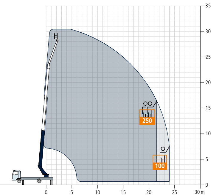
Drehbarer Korb PK 250-D, Tragfähigkeit von max. 250 kg
